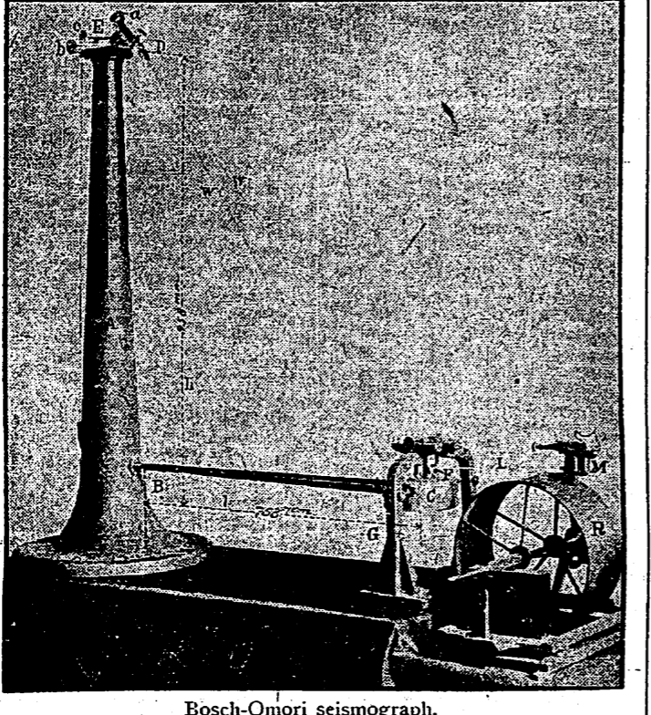
Bosch-Omori seismograph.
